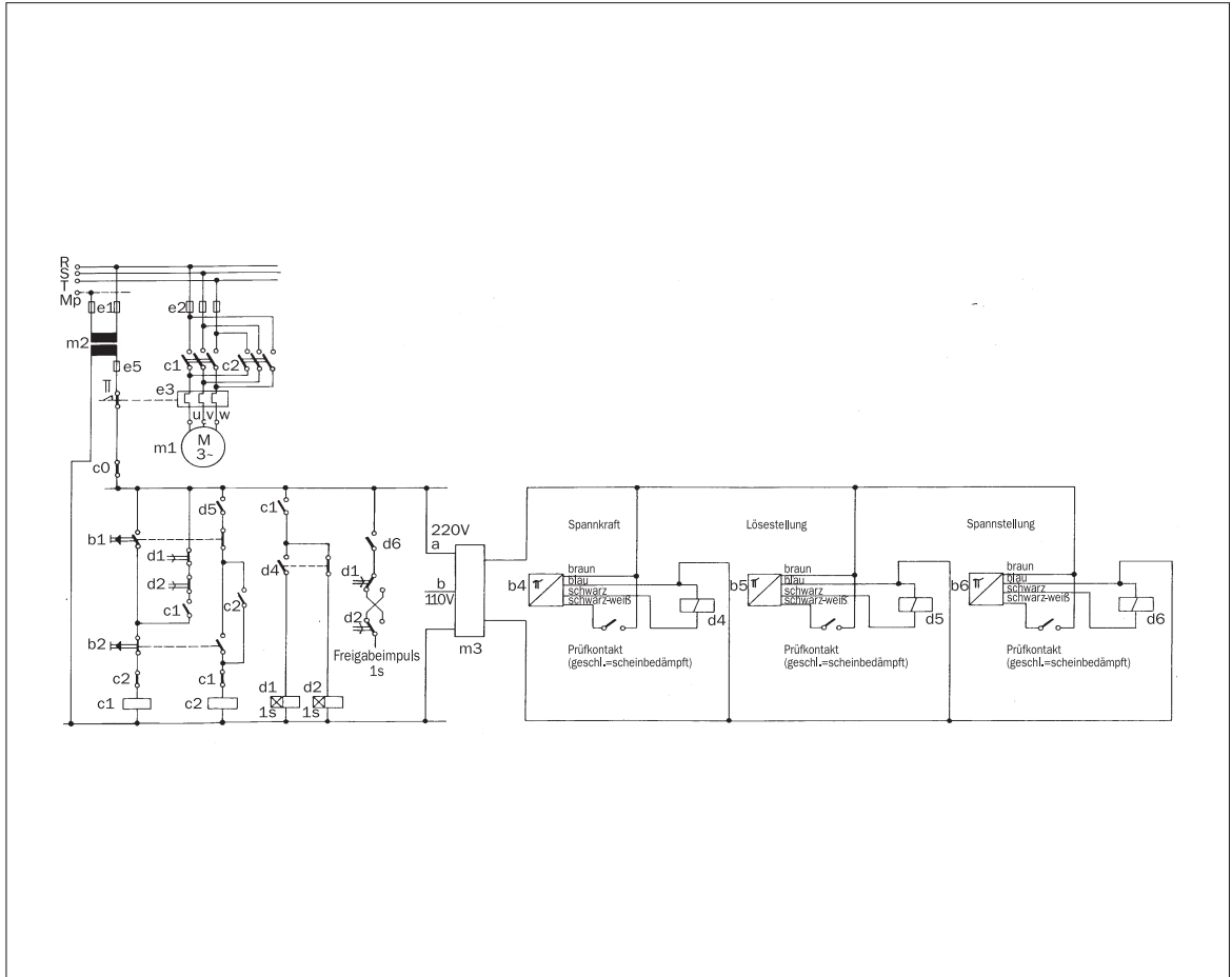
Prinzipschaltbild
